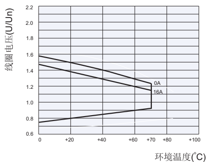
线圈工作温度曲线 (AC)
