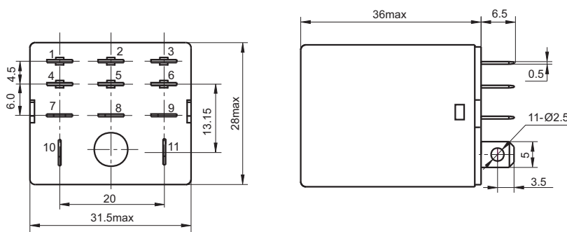
外形图
