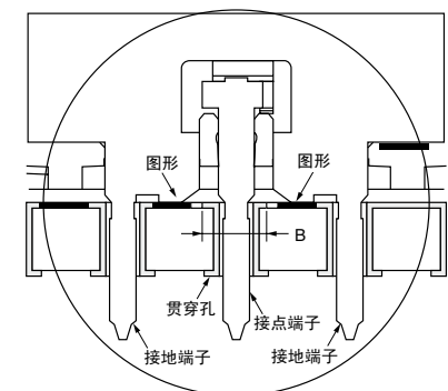
A部扩大断面图
