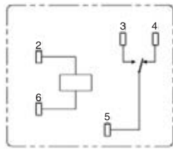
端子排列/外部接口 (BOTTOM VIEW)
