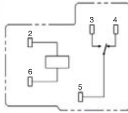
端子排列/外部接口 (BOTTOM VIEW)
